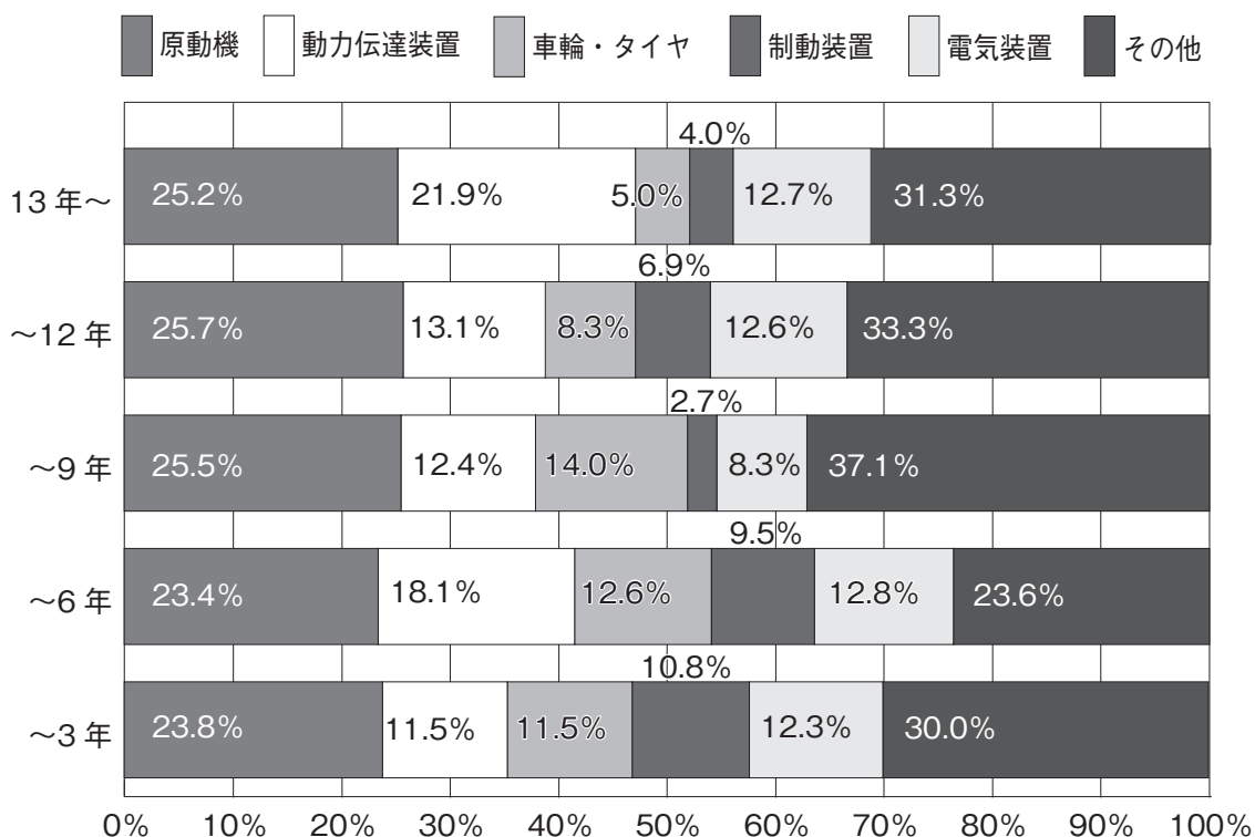
[図-2-6] 車齢別の故障箇所の状況 (令和3年)
