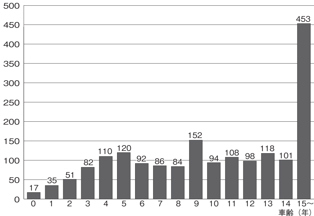
[ 図-2-2 ] バスの車齢別発生状況 (令和3年)
