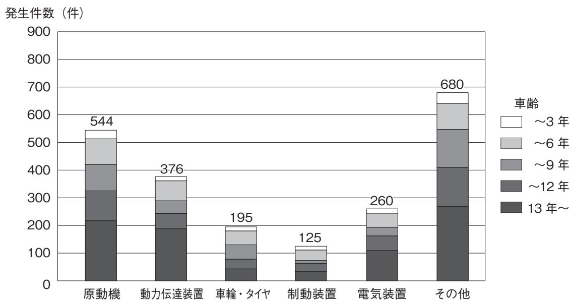
[図-2-5] 故障箇所の状況 (令和3年)
