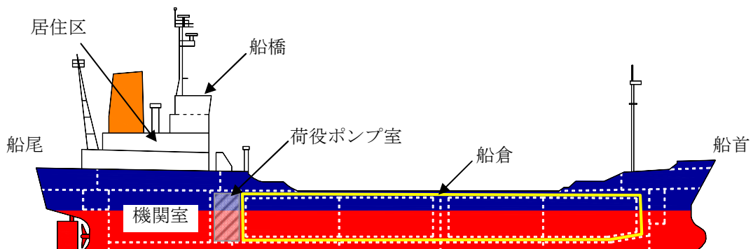
図 4-10 タンカー概観
