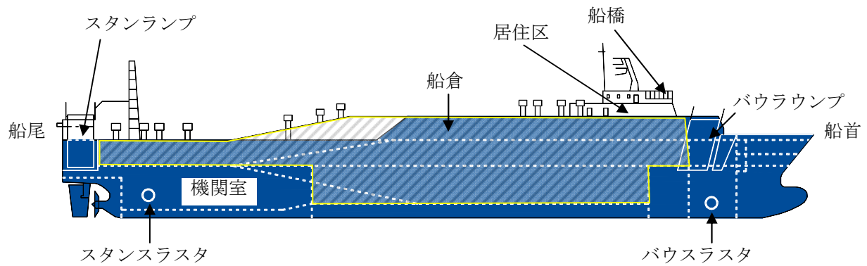
図 4-11 RORO船概観
