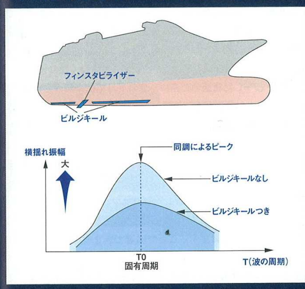
横揺れを抑えるビルジキールとフィンスタビライザー
