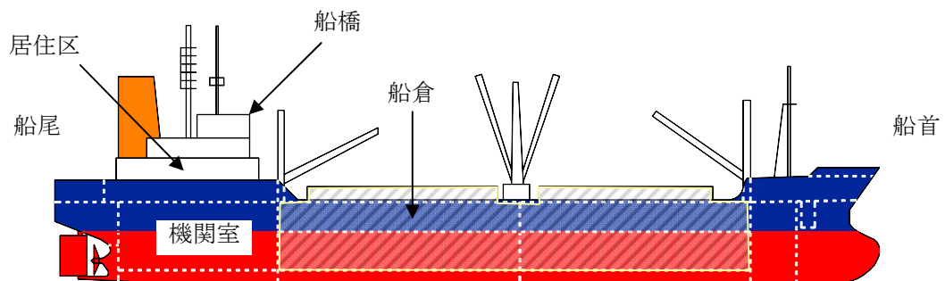
図 4-9 貨物船概観
