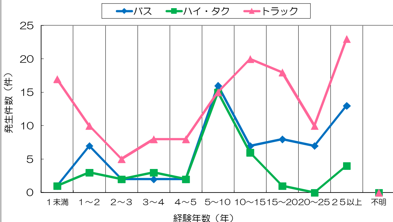
事故発生運転者の経験年数（運転者に起因するもの） （平成23年）
