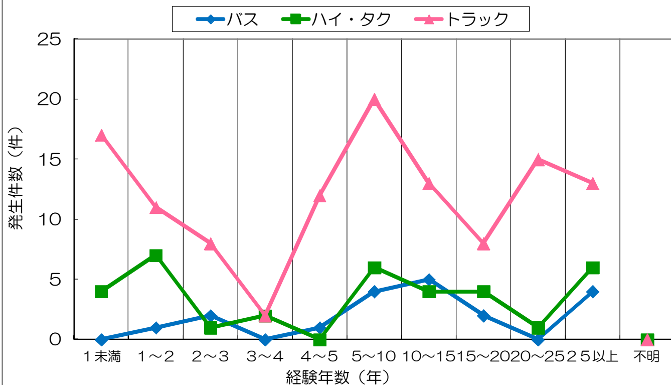
事故発生運転者の経験年数（運転者に起因するもの） （参考：平成22年）
