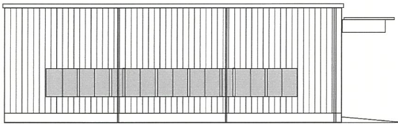
傾斜角上屋 南側立面図
