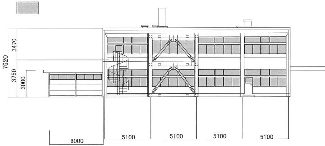
南側立面图
