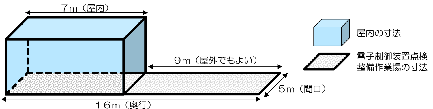
【電子制御装置点検整備作業場の寸法の概略図：普通自動車（大型）の例】
