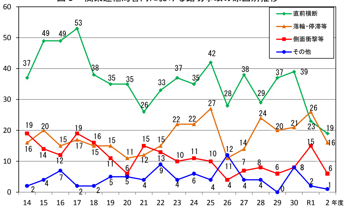
図5 関東運輸局管内における踏切事故の原因別推移
