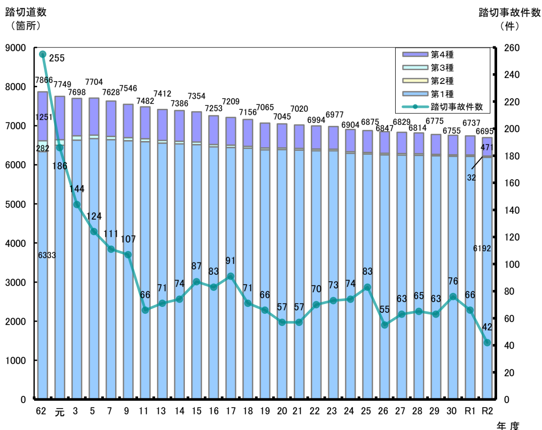
図6 関東運輸局管内における踏切道数と踏切事故件数の推移
