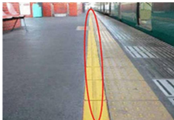
ホーム点字ブロック内方線
