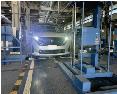
テスターによるヘッドライトの検査
