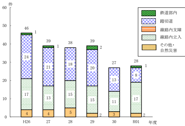
図-1 運転事故の原因別件数の推移
