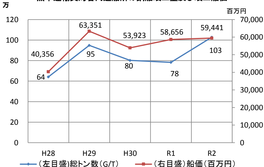
熊本運輸支局管内造船所の鋼船竣工量及び竣工船価
