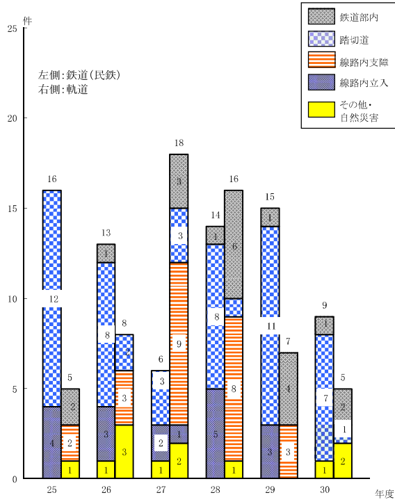
図一五 運転事故の原因別件数の推移
