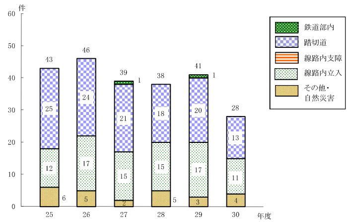
図一 1 運転事故の原因別件数の推移
