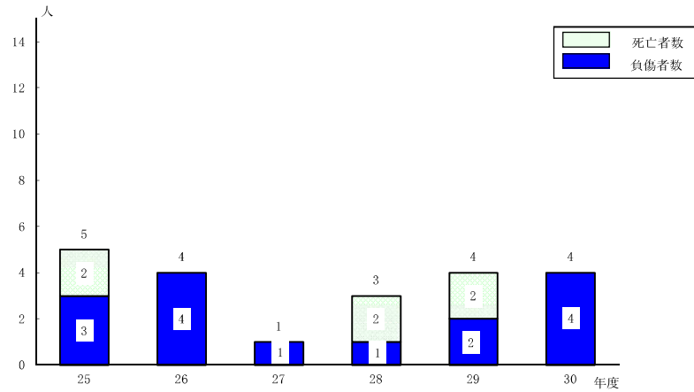
図一12 踏切障害事故 原因別件数の推移
