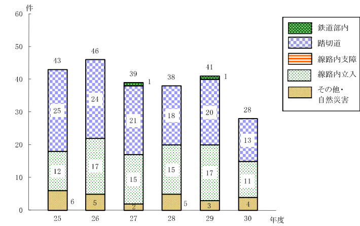
図一 1 運転事故の原因別件数の推移
