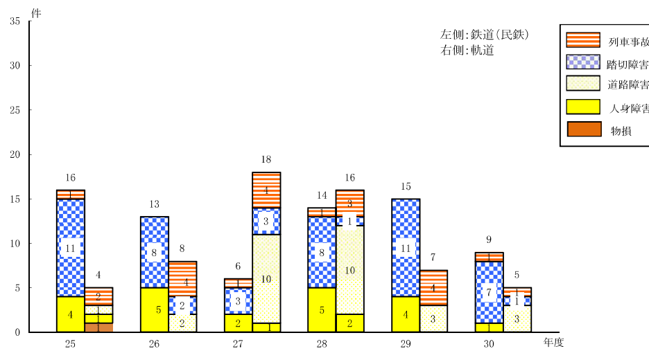
図三 運転事故の種類別件数の推移
