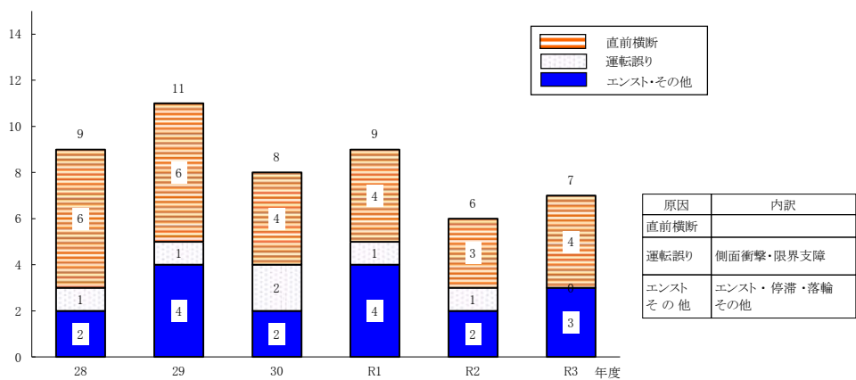
図-13 踏切障害事故 衝突物別件数の推移
