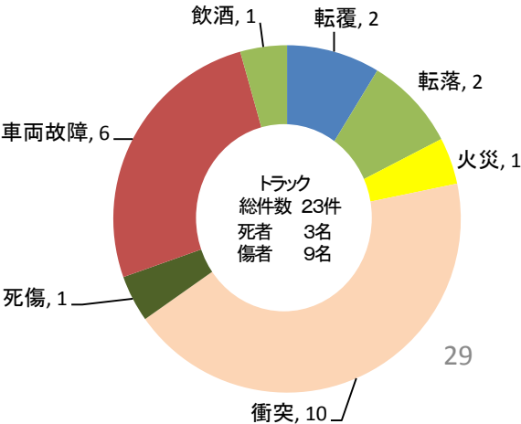
トラックの事故種別発生状況(令和2年度)
