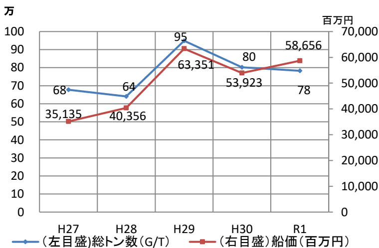
熊本運輸支局管内造船所の鋼船竣工量及び竣工船価
