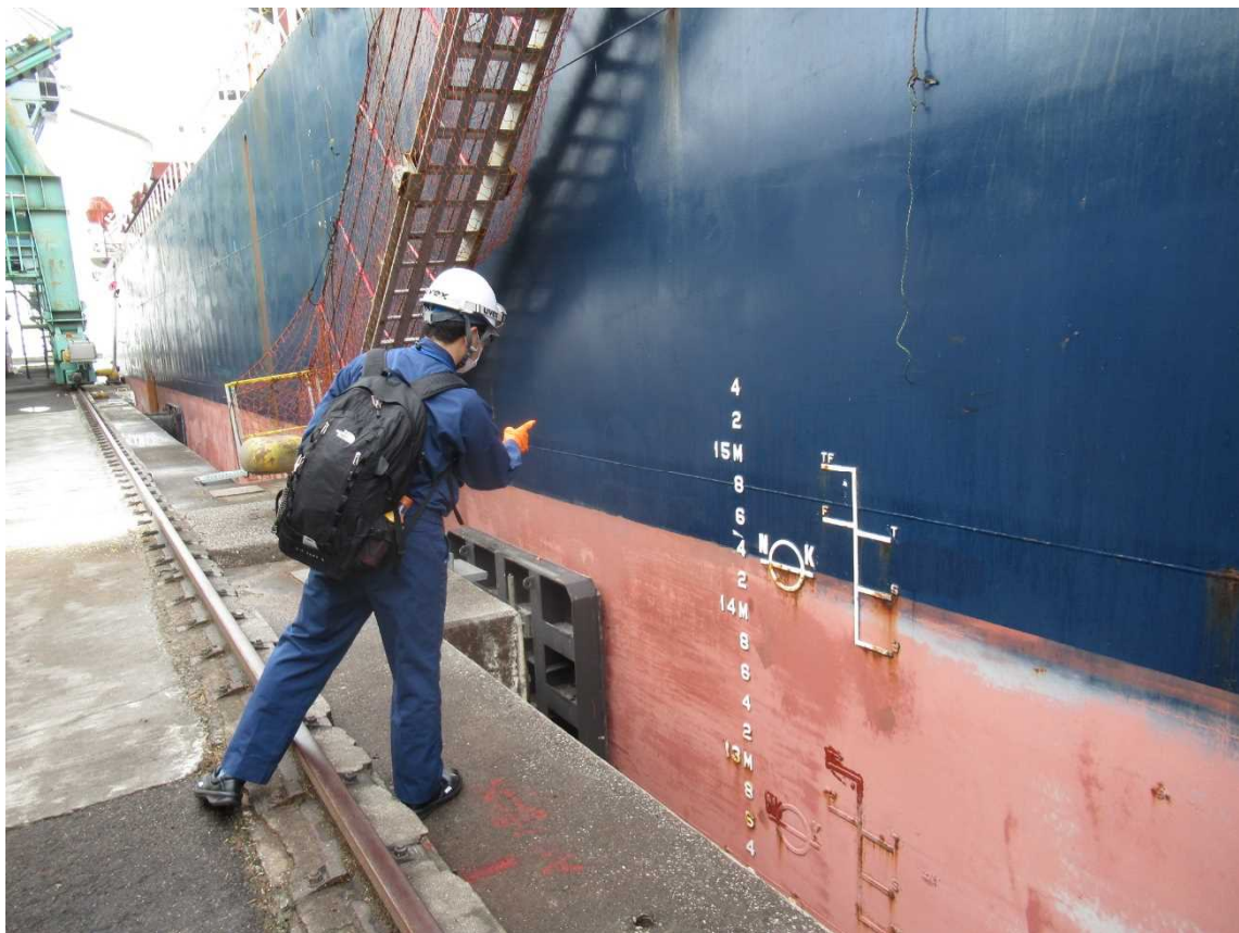
貨物船の満載喫水線を検査する外国船舶監督官
