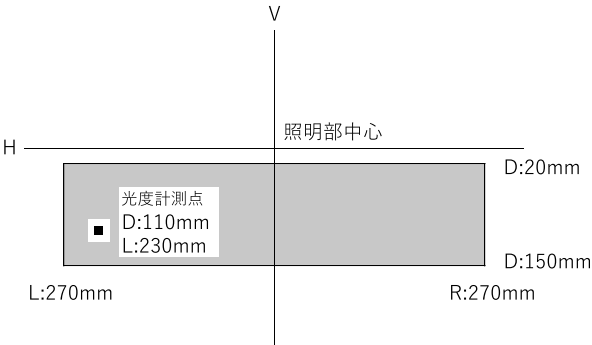
エルボ一点判定、照明部中心高さ 1メートル以下
