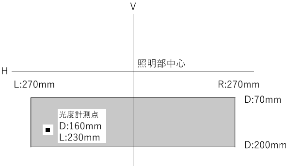
エルボ一点判定、照明部中心高さ 1メートル超え
