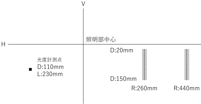
カットオフライン判定、照明部中心高さ 1メートル以下
