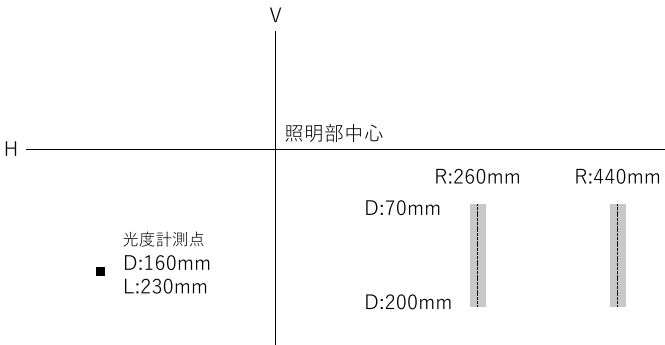
カットオフライン判定、照明部中心高さ 1メートル超え
