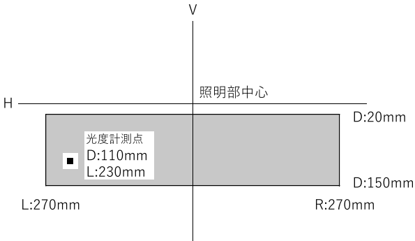
エルボー一点判定
