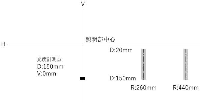
カットオフライン判定
