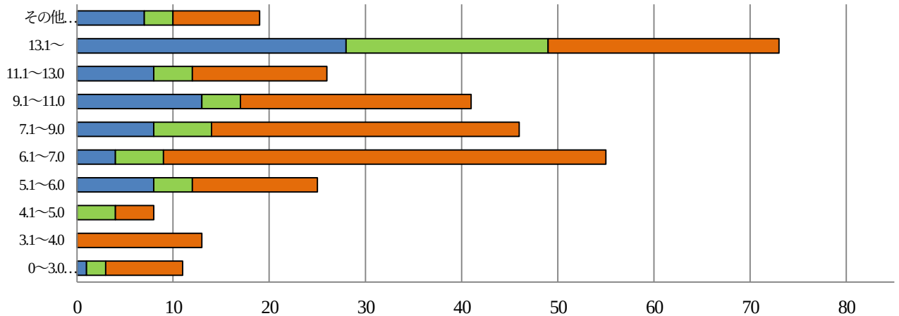
〔図17〕 道路幅員における事故発生状況（総件数 317件）
