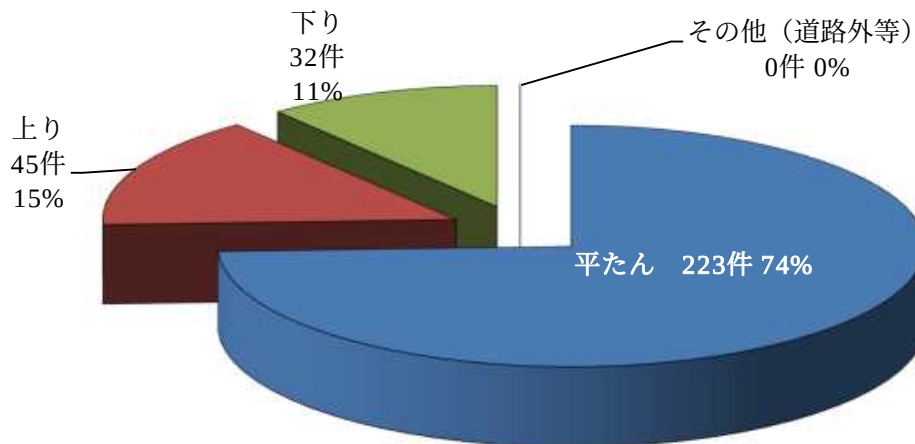
〔図18〕 道路の勾配等における事故発生状況（総件数 300件）
