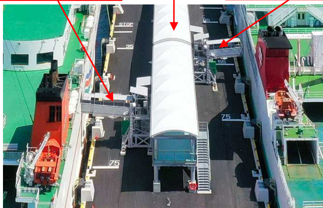
スロープとフェリーの乗降口 バリアフリータラップはフェリー会社が設置
