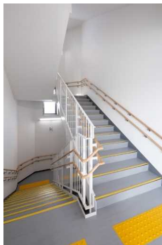
主階段 (2段手摺、点字表示)
